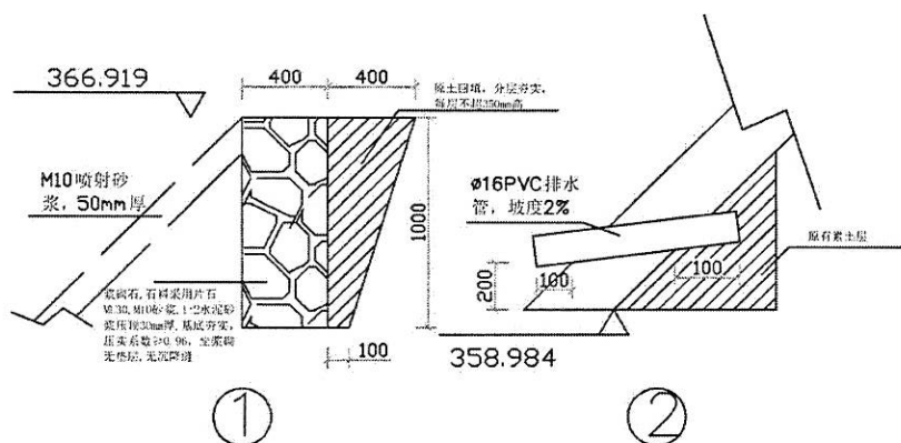
滑坡区域立面图
